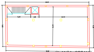
PLANTA SOTANO
