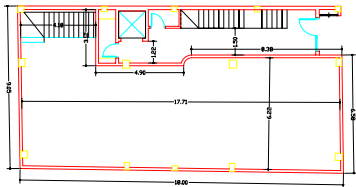
PLANTA BAJA
